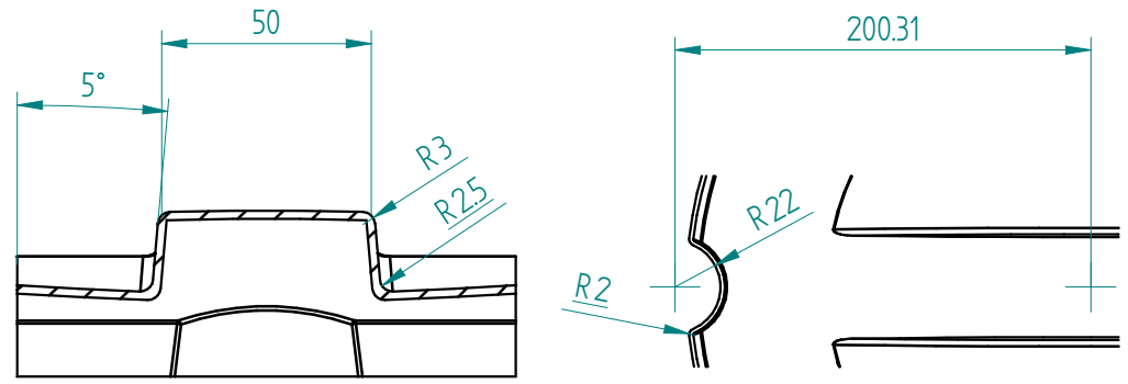
DOORSNEDE C-C
