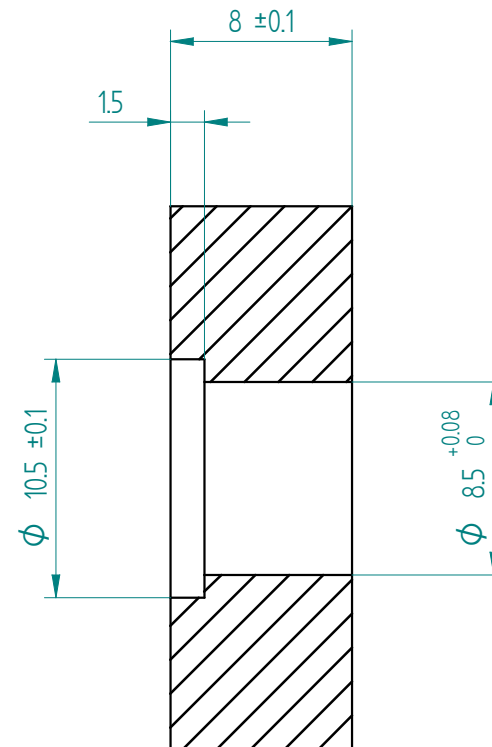
DOORSNEDE A-A
